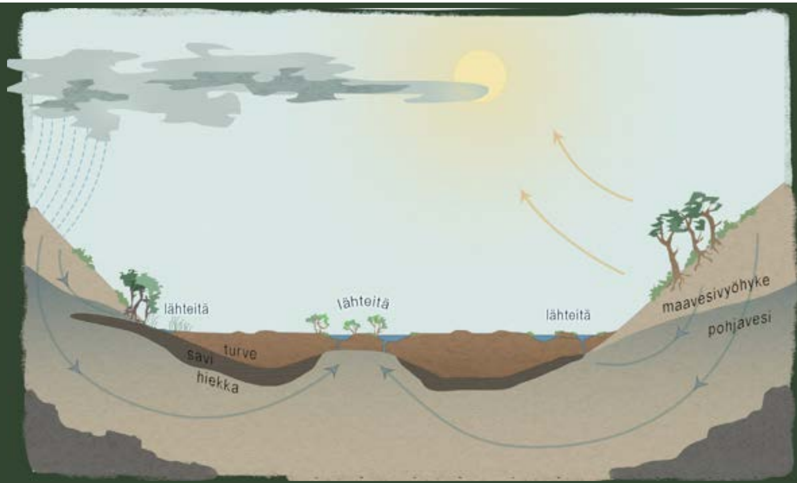
Piirros 1. Pohjaveden ja lähteiden muodostuminen. Keväiset sulamisvedet ja sadevesi vajoaa pohjavesimuodostumaan maavesivyöhykkeen läpi. Maaston muodot ja maaperän maalajin sekä lajittuneisuuden muutokset vaikuttavat siihen, missä pohjavesi purkautuu maanpinnalle muodostaen lähteitä.
