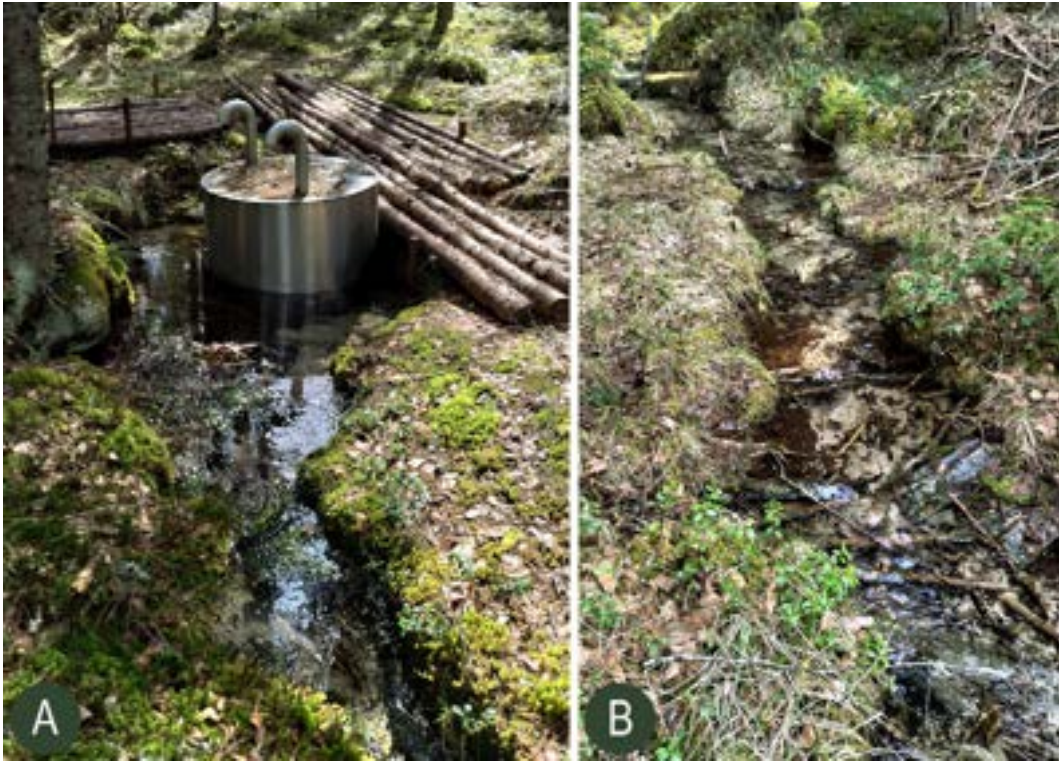
Kuva 76. A) Hiekkapohjaisen lähteen laidalle on tehty puurimoista kulkureitit ja lähteeseen on asennettu rosterinen lähdekaivo. Pohjavesi purkautuu lähdekaivon sisään ja sieltä kolmesta ylivuotoaukosta vuolaasti virraten allikkoon. Kaivon vesitalouteen kohdistuvat haitat ovat vähäisiä ja vesi on allikossa jatkuvassa liikkeessä. Allikkolähteellä ei ole varsinaista ennallistamistarvetta ja se on muutoinkin edelleen vedenottokäytössä. Kaivosta johtuen lähde ei kuitenkaan saa metsälain mukaista suojaa. Kun vedenotto päättyy, rosterinen kaivopönttö voidaan nostaa käsivoimin pois lähteestä. B) Allikkolähteestä alkunsa saava lähdenoro on aikanaan perattu, mutta palautunut luonnontilaisen kaltaiseksi.
